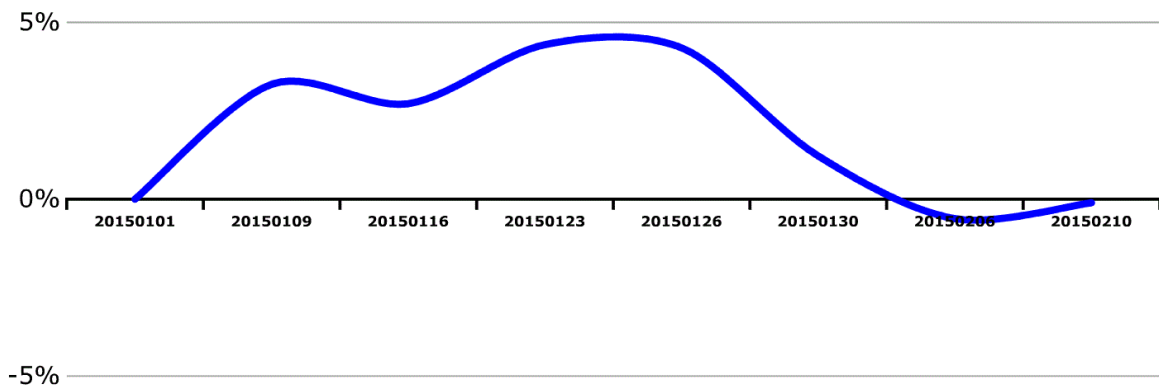
达摩掌2015年的累积收益曲线 (激进型)
