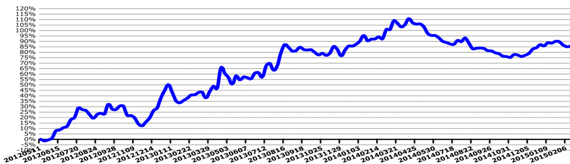
达摩掌的累积收益曲线 (激进型)
